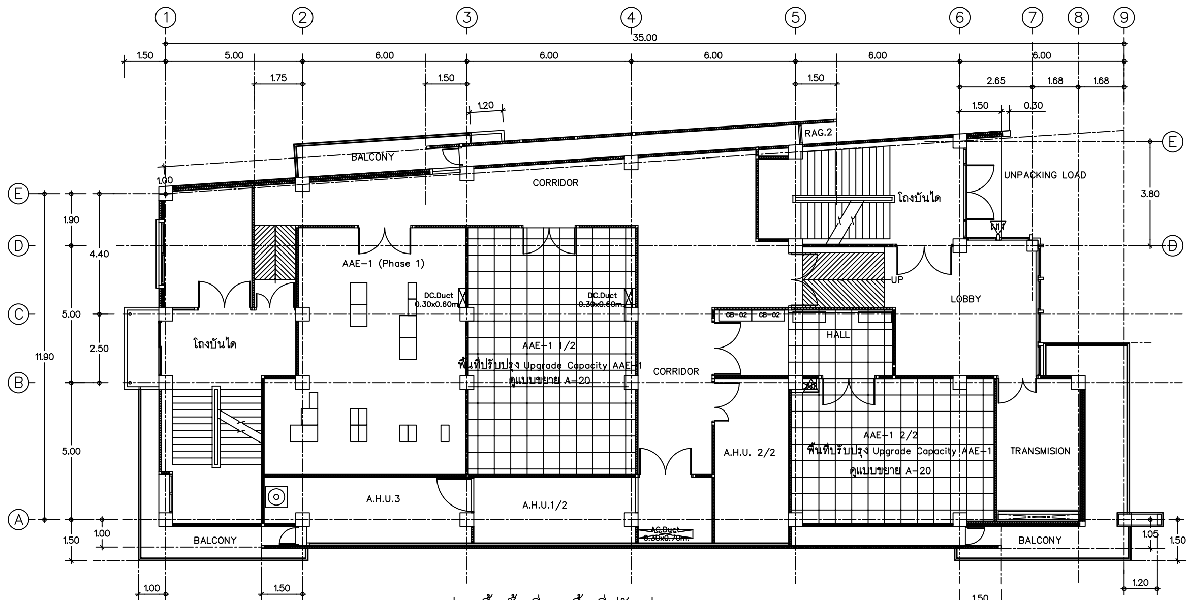
แปลนพื้นที่ 4 พื้นที่ปรับปรุง Upgrade Capacity AAE-1 มาตราส่วน 1 : 125
