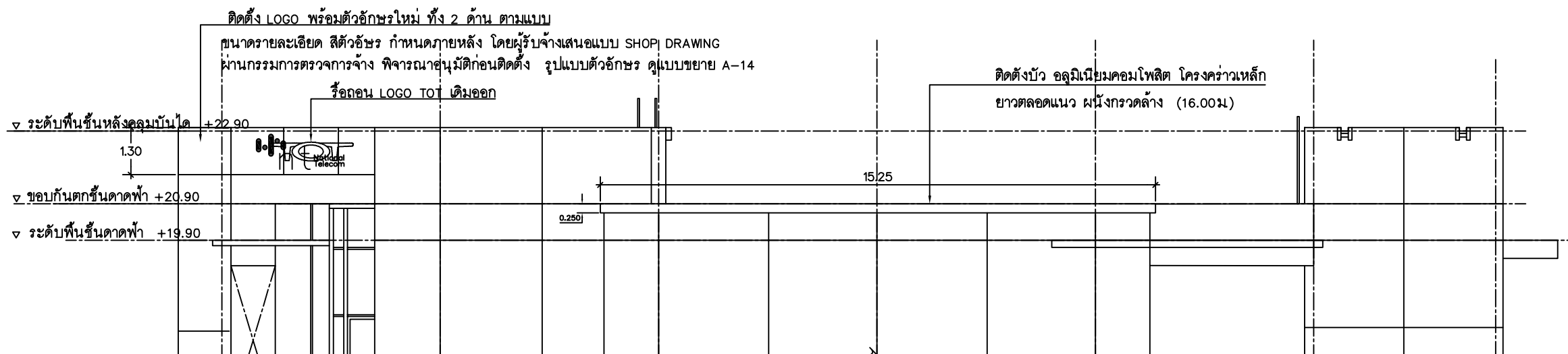
แสดงรูปด้านข้าง ทิศตะวันออก มาตราส่วน 1 : 125
